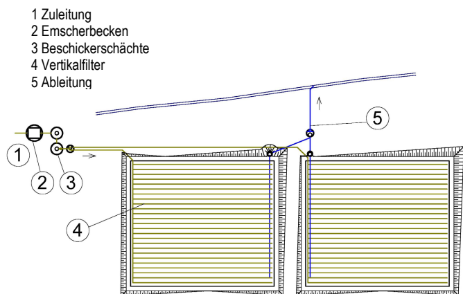
Übersichtsplan der Kläranlage Dorweiler - Draufsicht
